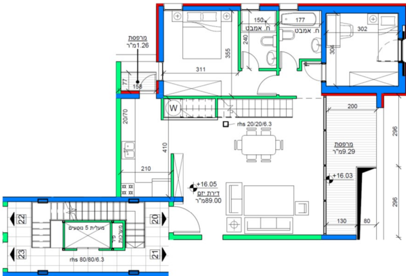
תוכנית קומה ה - תמא 2 +16.05 1 : 100
